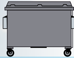
Rolcontainer kunststof en staal 1100 liter L 121 x B 102 x H 120 cm
