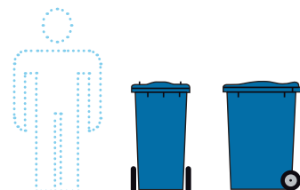
Rolcontainer kunststof 240 liter L 58 x B 65 x H 104 cm
